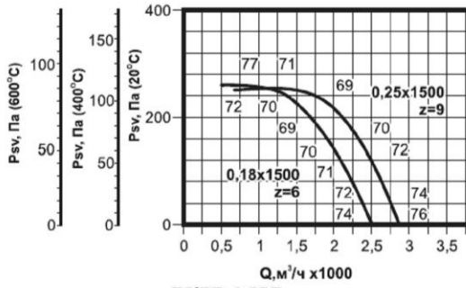
ВКРВ-3,55Ду
