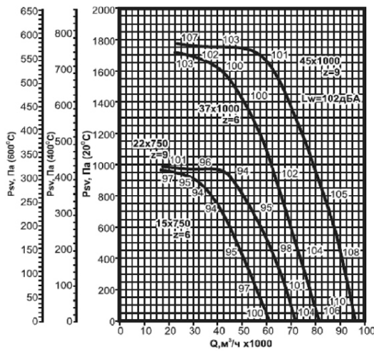
BKPB-12,5Дy
