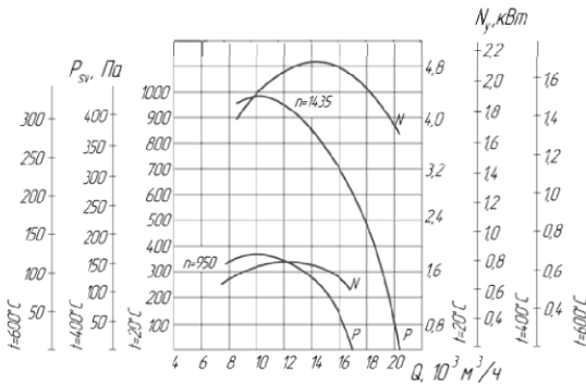
ВКРМ-6,3Ду
