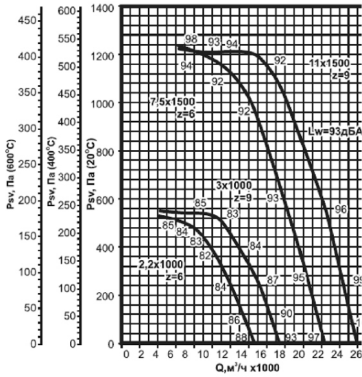
BKPB-7,1Дy
