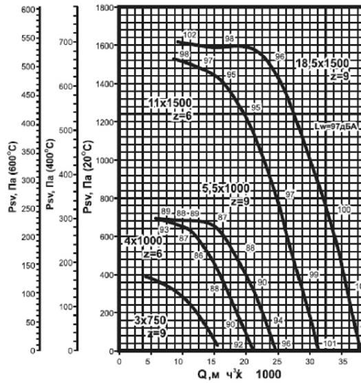
BKPB-8Дy
