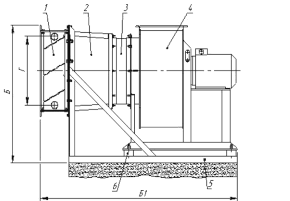
Агрегат вентиляционно-приточный АВП 60/3000, АВП 75/3000, АВП 100/5000, АВП 160/10000, АВП 400/3000
