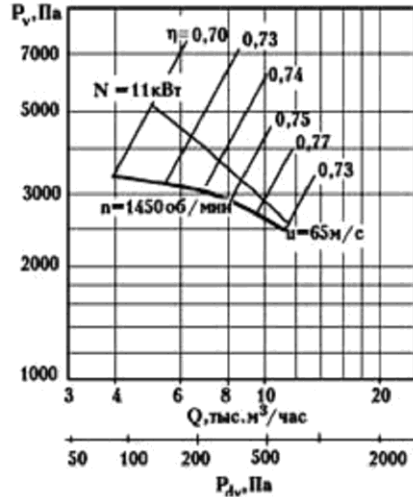
ВЦ5-35-8,5
