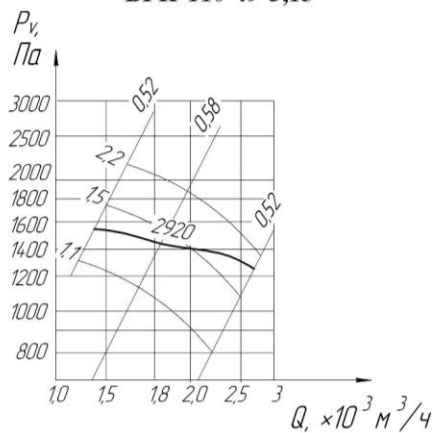
ВРП-110-49-3,15
