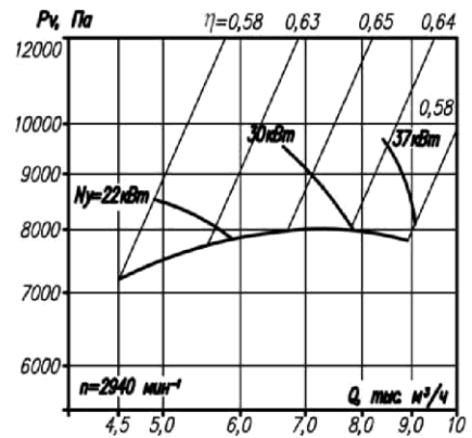
ВР-12-26-5
