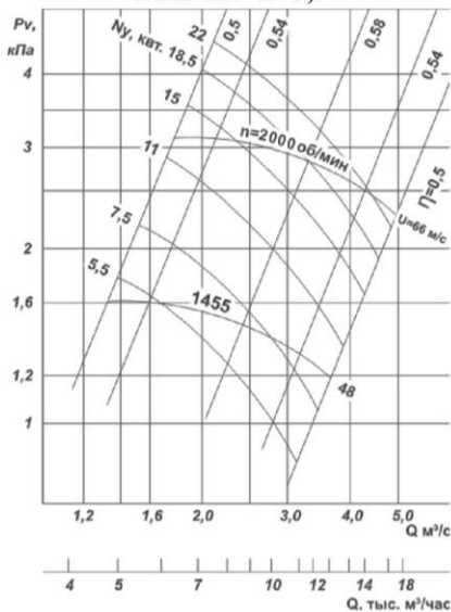
ВРП-110-49-6,3
