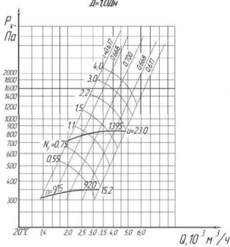
ВЦ 14-46-3,15
