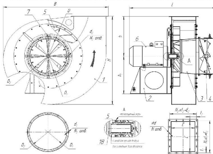
1-карлус, 2-пань 3-патрубок вьсаыбывающй, 4-апарат нагрывающй, 5-колесо рабоче, 6-электродвигатель, 7-фиксатор
