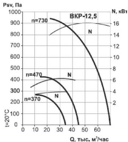
БКРМ-12,5
