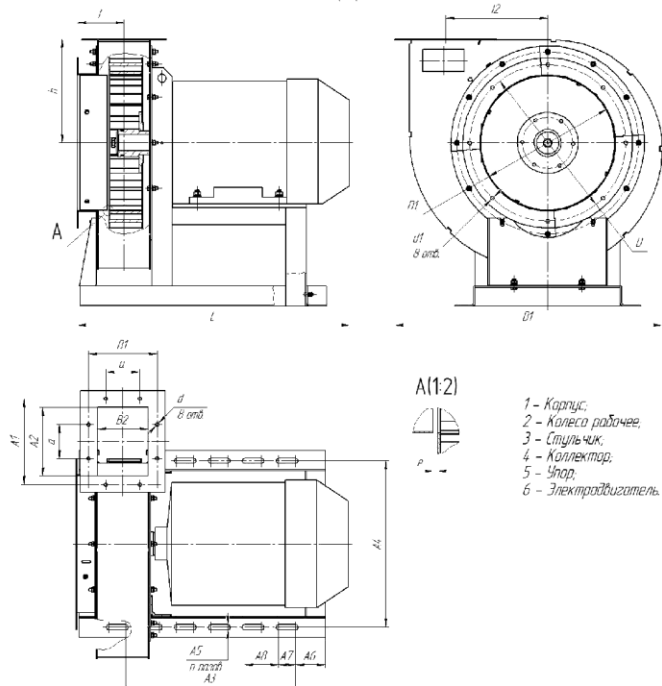
Габаритные и присоединительные размеры в мм
