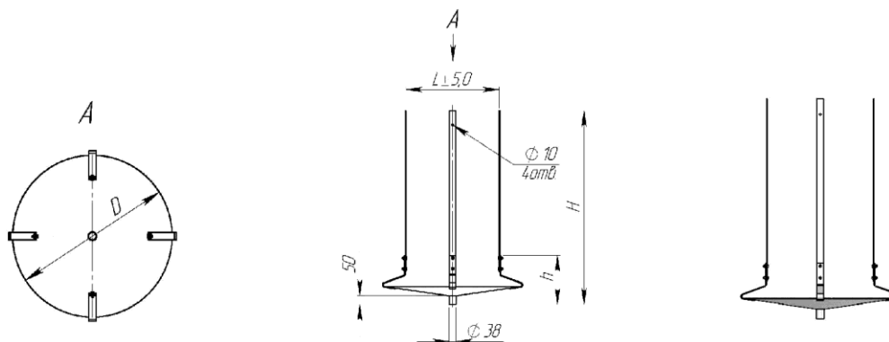
Размеры, мм
