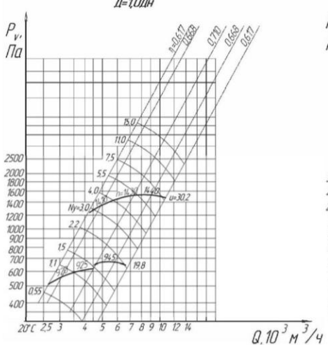
ВЦ 14-46-5
