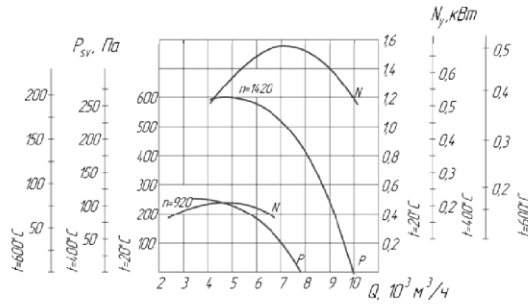
ВКРМ-5Ду
