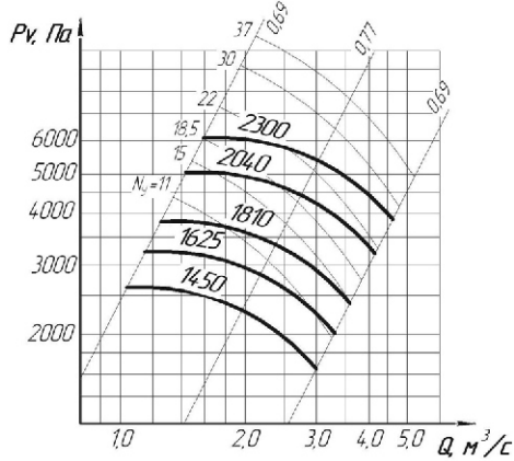
ВР-132-30-8
