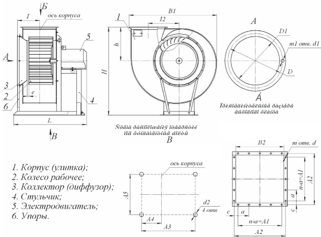
Габаритные и присоединительные размеры в мм
