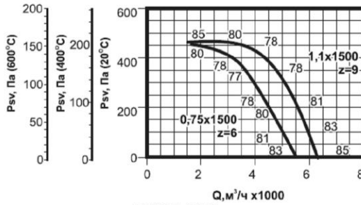
ВКРВ-4,5Ду
