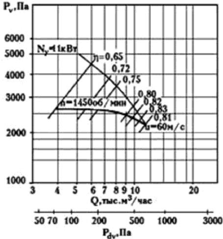
ВЦ5-45-8
