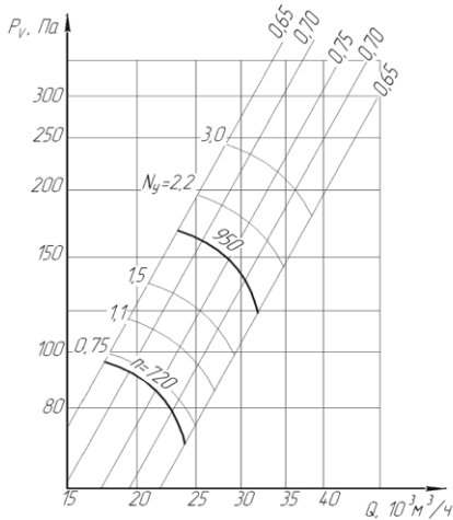
ВО-06-300-10
