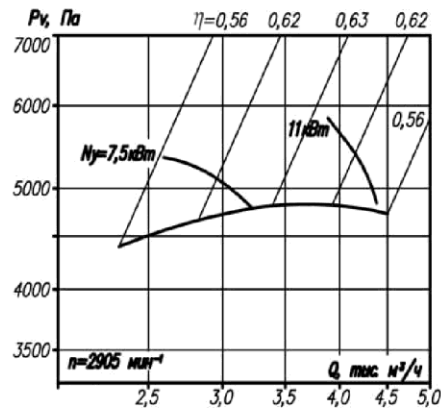
ВР-12-26-4
