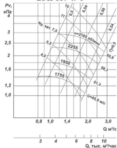
ВРП-110-49-10
