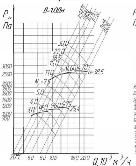
ВЦ 14-46-5
