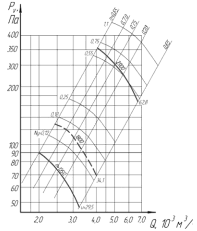
ВО-06-300-4
