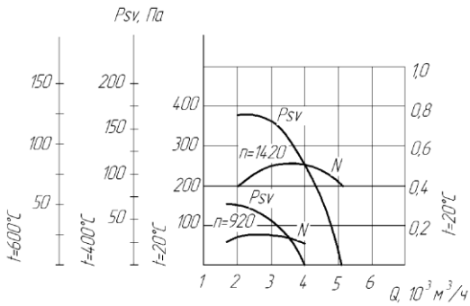
ВКРМ-4Ду
