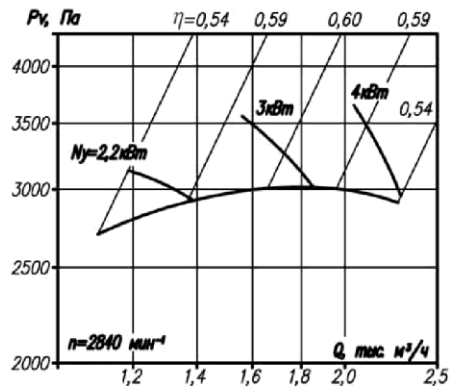
ВР-12-26-3,15
