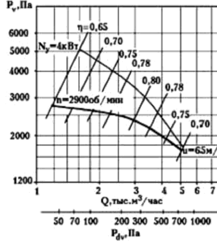
ВЦ5-45-4,25
