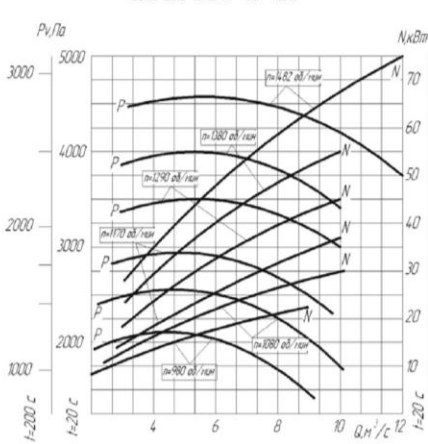
ВРП-110-49-10
