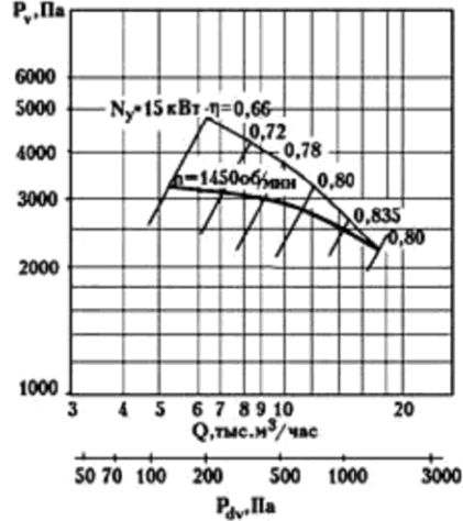
ВЦ5-45-8,5
