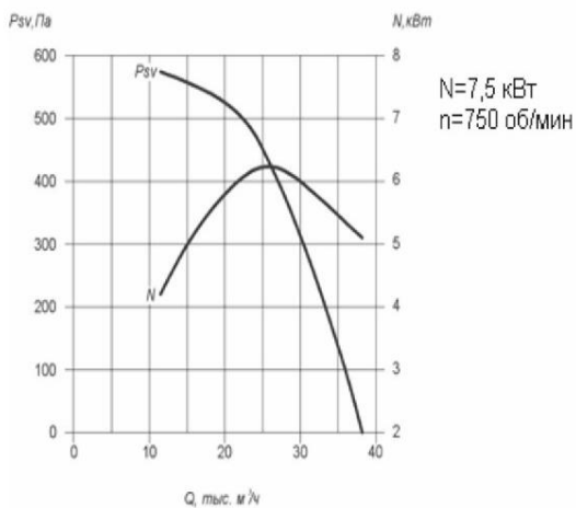
БКРМ-10
