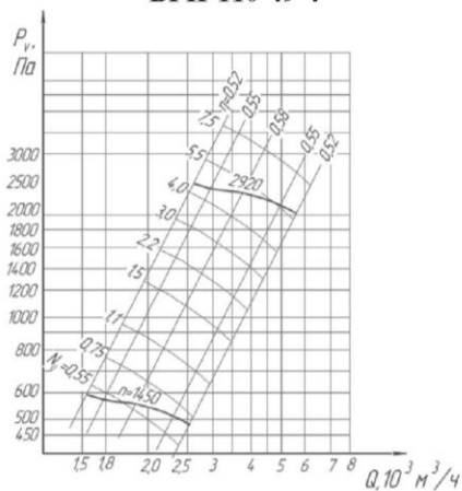
ВРП-110-49-4
