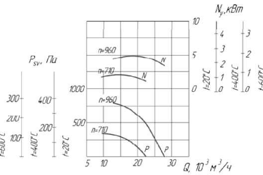
ВКРМ-8Ду
