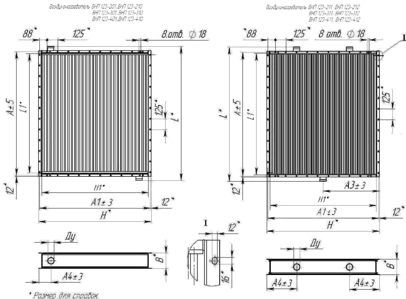
Рисунок 1 Габаритные и присоединительные размеры
