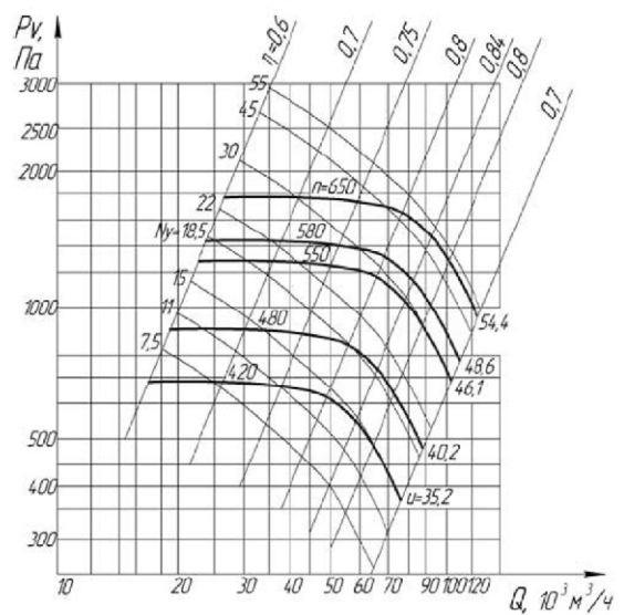
ВЦ4-76-16
