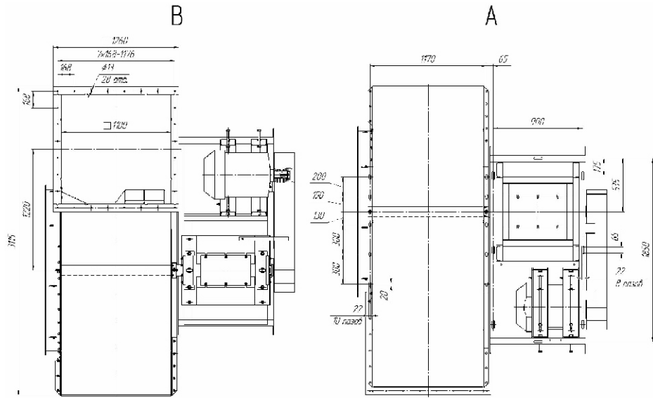
ВЦ4-70-16
