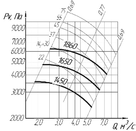
ВР-132-30-10
