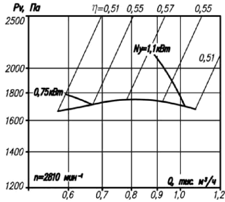
ВР-12-26-2,5
