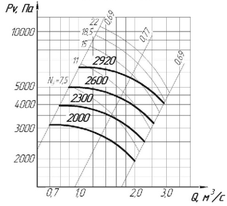
ВР-132-30-6,3
